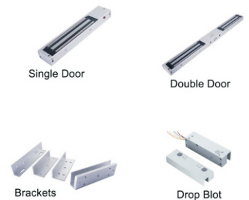
EM LOCK & ACCESSORIES CS-AD-EL61/62 CS-AD-LB612 / CS-DB63
